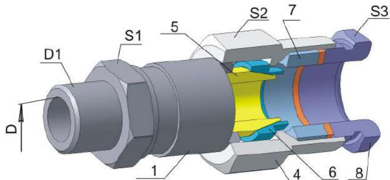
Рисунок 4.3 - Конструкция кабельного ввода для монтажа бронированного кабеля
